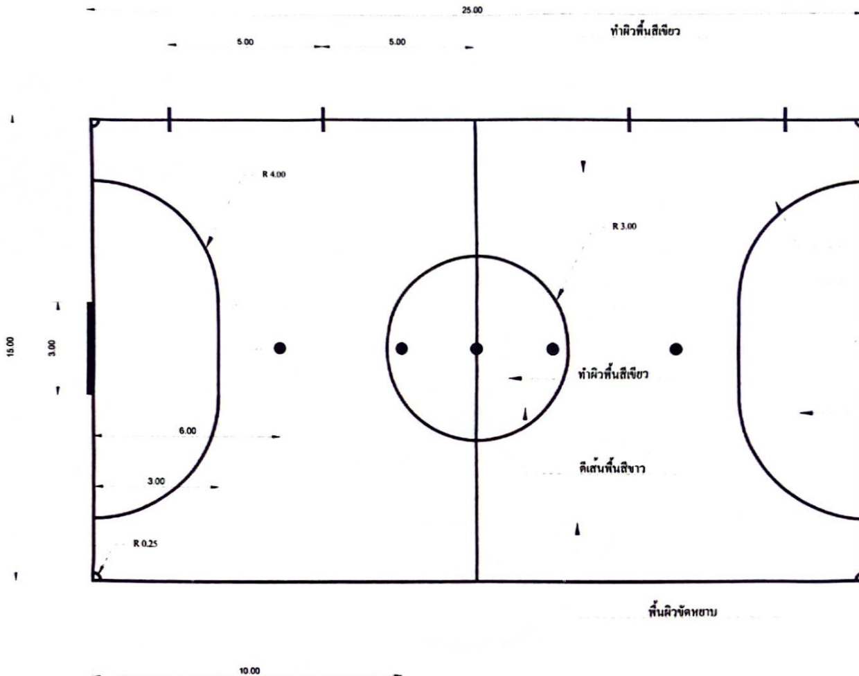
แบบสนามฟุตซอล ฟุตบอล 5 คน
